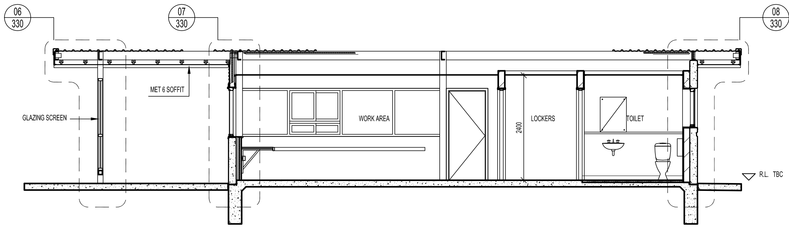
04 SECTION 1:50
