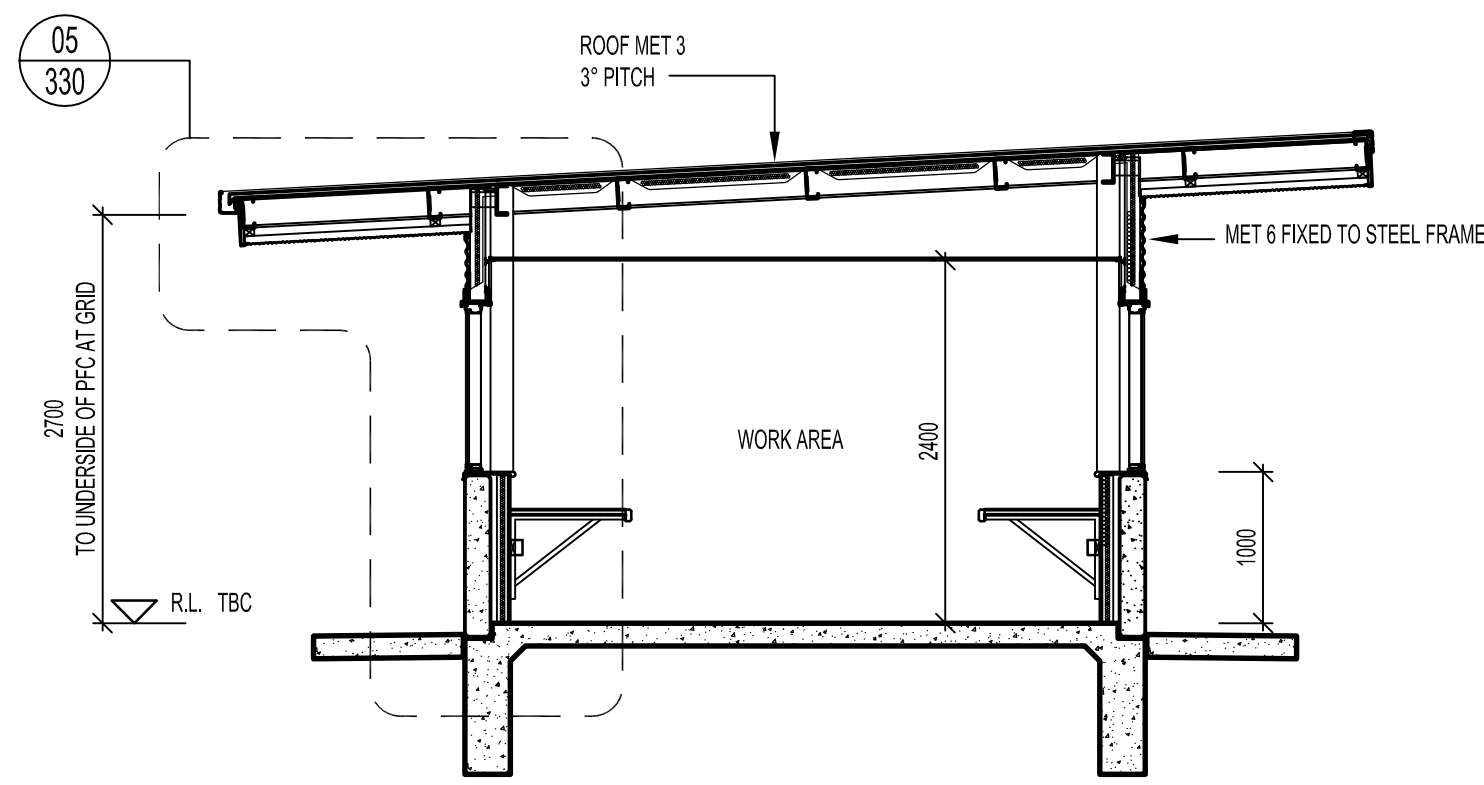
05 SECTION 1:50
